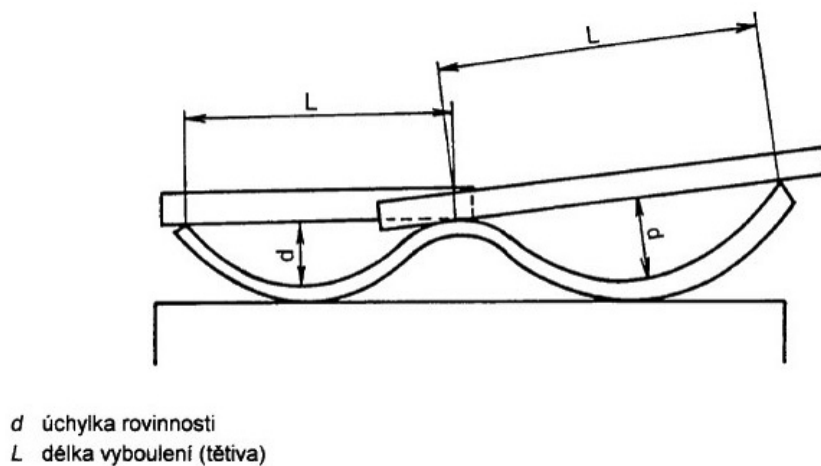
Obrázek 2: Vyboulení
