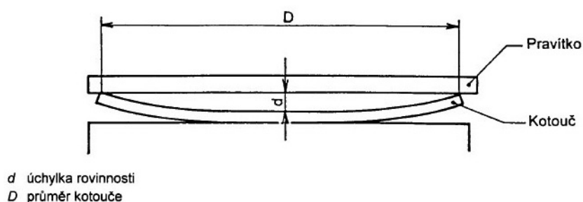
Obrázek 1: Klenutí
